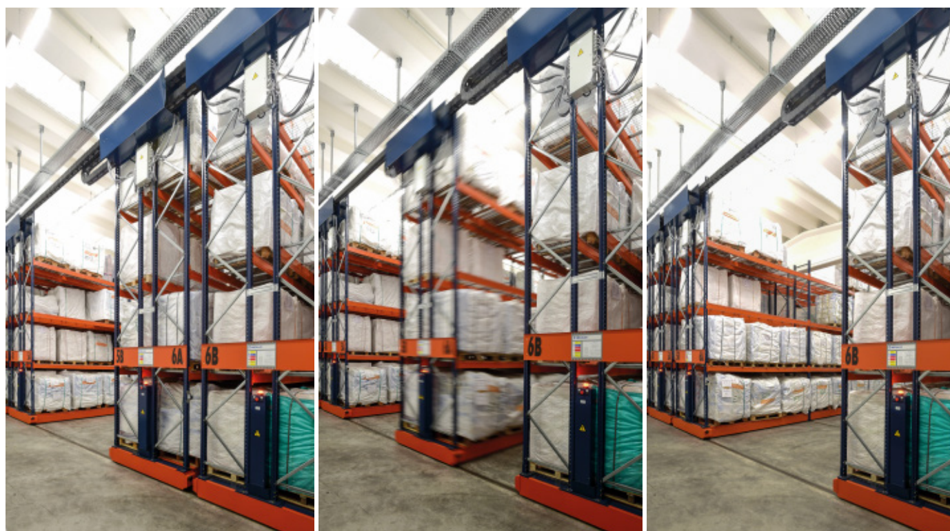
Images illustrant le fonctionnement du système de rayonnages sur bases mobiles Movirack
